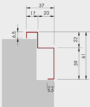
Detalle marco
